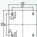
壁面設置金具(穴寸法図)
