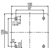
壁面設置金具(穴寸法図)
